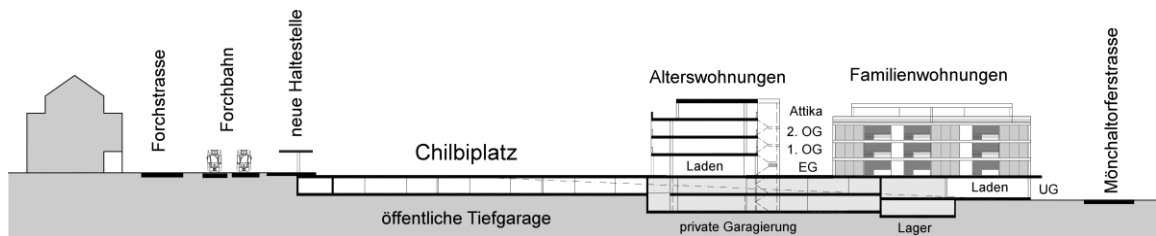
Schnitt von der Forchstrasse zur Mönchaltorferstrasse mit neuem Chilbiplatz und angrenzender Überbauung mit Läden und Wohnungen
